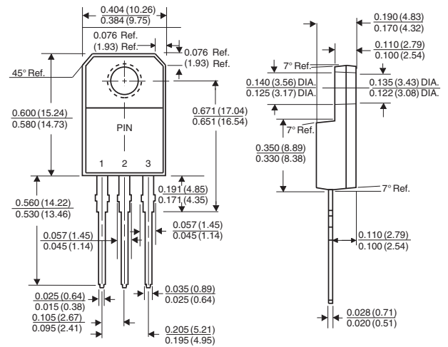
ITO-220AB
