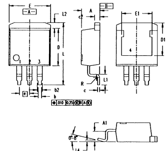
TO-263 AA Outline
